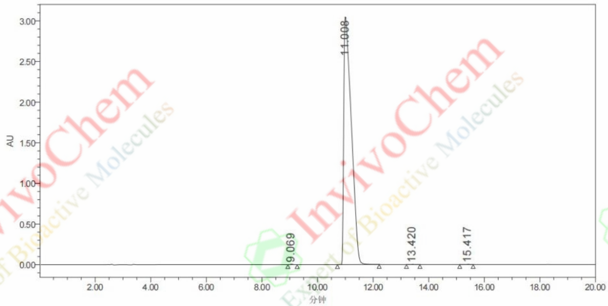
色谱峰结果
