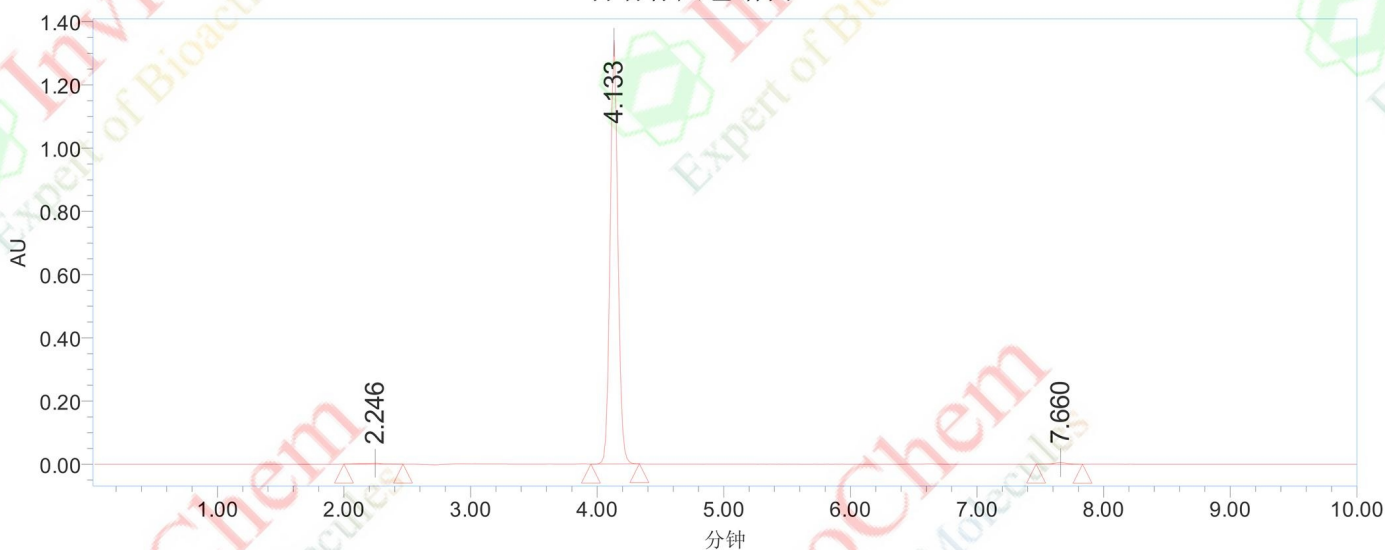
自动标尺色谱图
